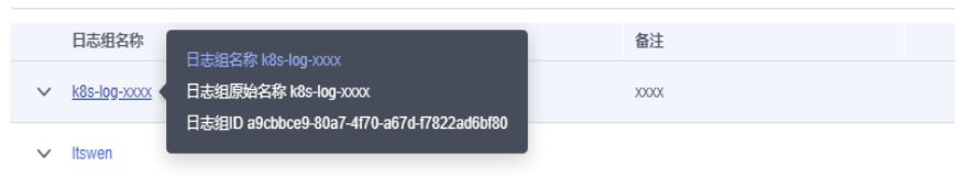
图 4-11 日志组名称
