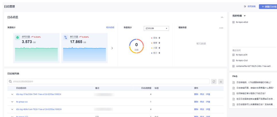
图 4-1 控制台首页
