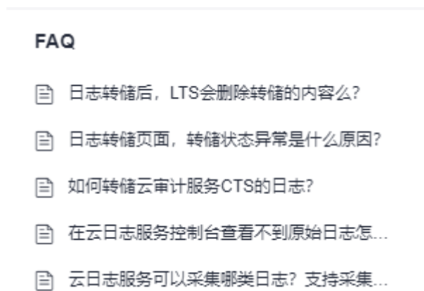
图 4-7 FAQ
