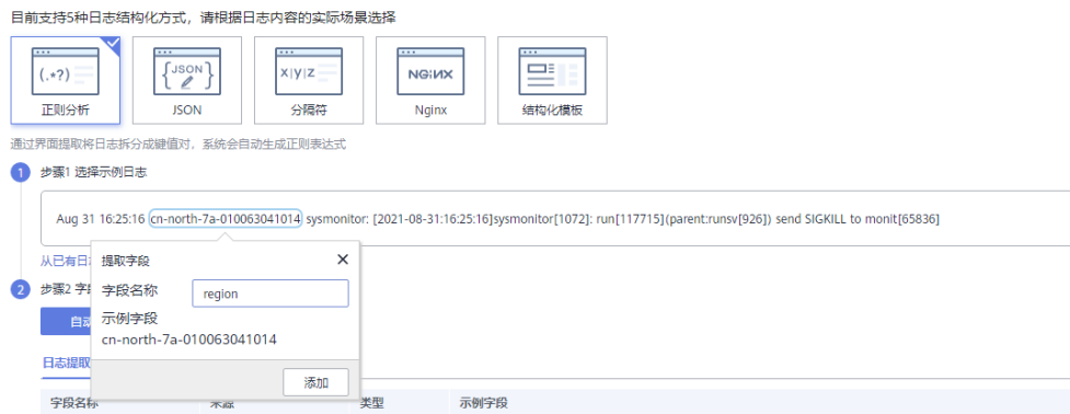
图 7-3 选择字段
