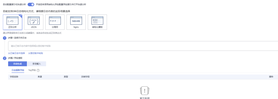
图 7-2 日志结构化
